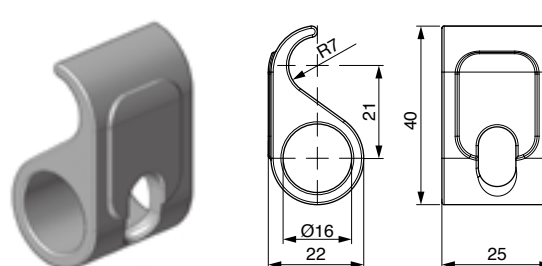
PALETTA IN FUSIONE - LOCKING PLATE
