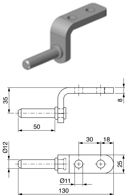
PERNO RIBATTUTO ZINCATO Ø12 ZINC PLATED PIN Ø12
